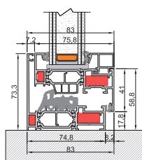
Nodo Inferiore Telaio L
